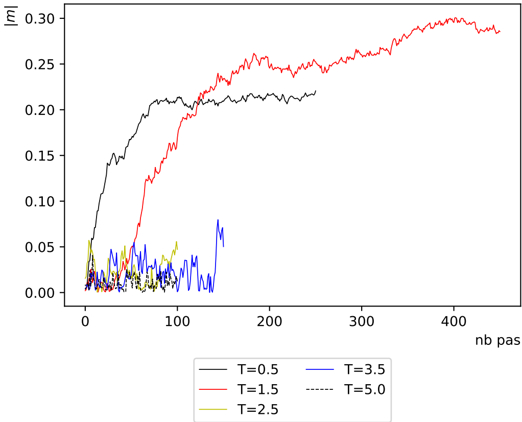
Evolution de l'aimantation sur critère Estimation par intervalle, N=128
